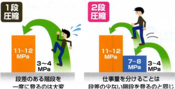
2段圧縮ロータリー CO 2 コンプレッサー
